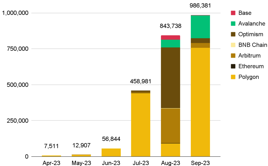
Hình 5: Tổng số giao dịch tài khoản thông minh ERC-4337 tăng dần qua từng tháng
